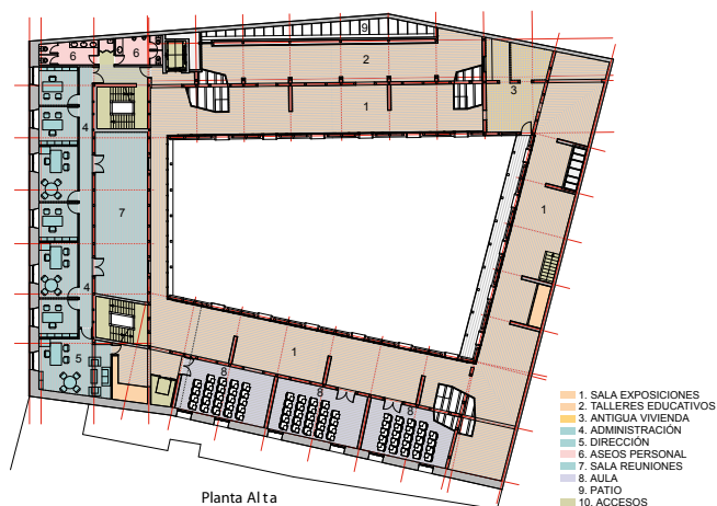
Planta Alta
