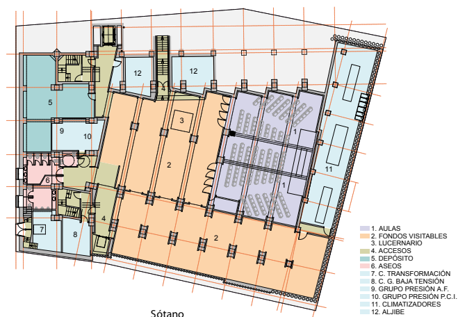
Sótano
