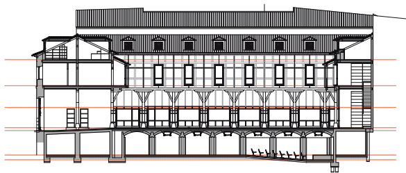
Sección Longitudinal
