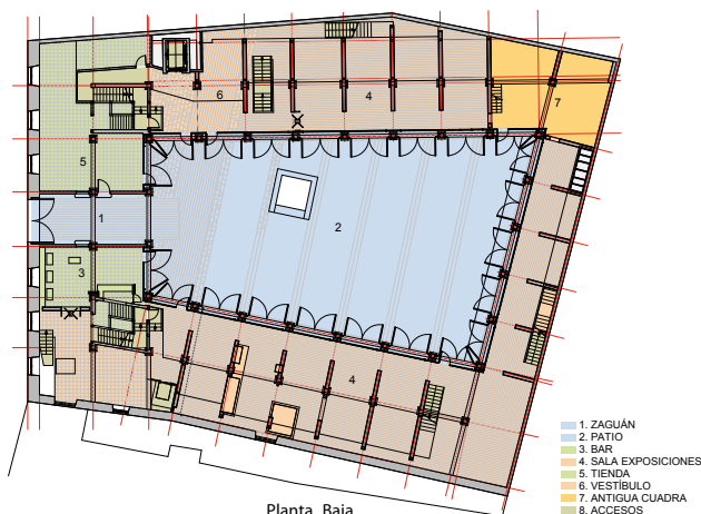
Planta Baja
