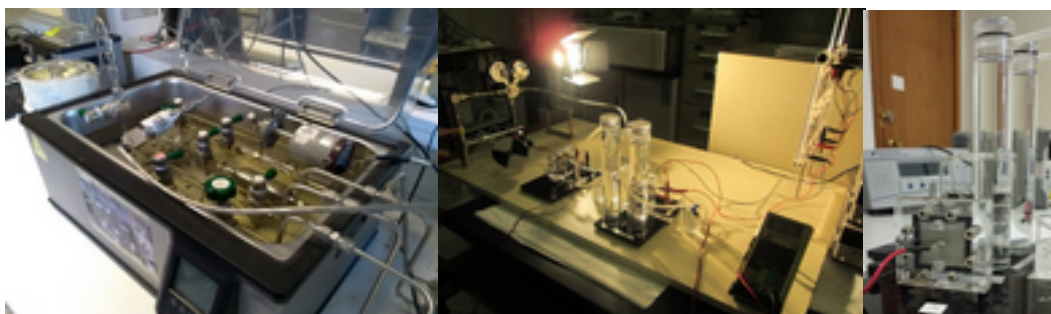
Fig.5. Imagen de varios de los sistemas del laboratorio que usan los estudiantes en la asignatura de hidrógeno. De izq. a dcha. Sistema Sieverts de hidrogenación; Sistema solar-hidrógeno, pila de combustible con electrolizador y detector de hidrógeno
