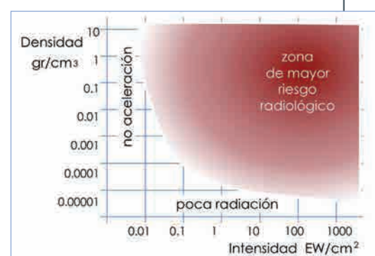
Figura 1. Esquema de la región de riesgo radiológico en función de los dos parámetros más relevantes: la intensidad del láser (con longitud de onda de 800 nanómetros) y la densidad del medio sobre el que se focaliza. Es evidente que si el blanco es de densidad muy baja apenas hay átomos con los que interaccione en el volumen focal y por ello no se genera radiación. La escala horizontal está en exavatios ( 10^{17} \text{ W} ) por \text{cm}^2 .
